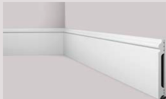
FL17 WALLSTYL® 170 x 18 x 2000 mm
